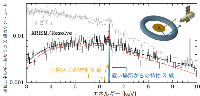
図1：Resolve と過去の X 線天文衛星「すざく」の X 線スペクトル（それぞれ、黒と灰色のクロスで表されている）。エネルギー 6 keV あたりで、遠く比較的ゆっくりと動いているガスからの細い特性 X 線（青線）に加え、ブラックホール近くの円盤からの広がった成分（オレンジ線）が、Resolve によって綺麗に見分けられていることがわかる。右上では、ブラックホール近傍から出た X 線が円盤や遠方のガスに当たり、特性 X 線が出るパスを示している。
