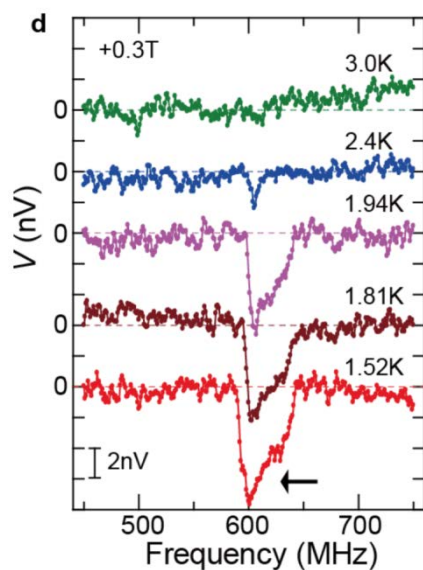
図 2. 観測されたスピンプンピング信号。核磁気共鳴によって核スピン波が励起される周波数 600MHz あたりに、2.4K 以下から電圧信号が確認できる。
